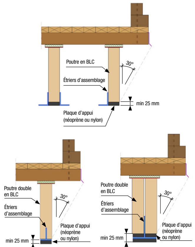
FIGURE 45 - Exemples d'appuis surélevés
