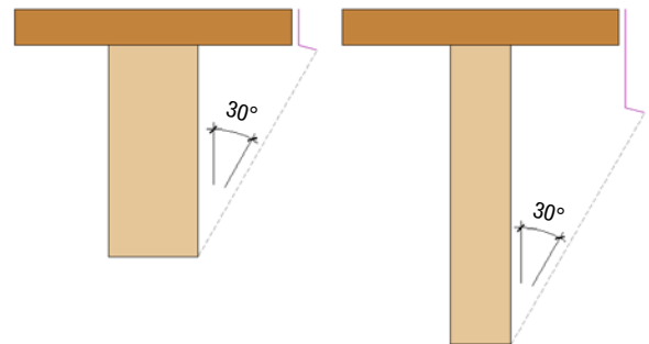
FIGURE 9 - Protection contre la pluie respectant un angle de 30°
