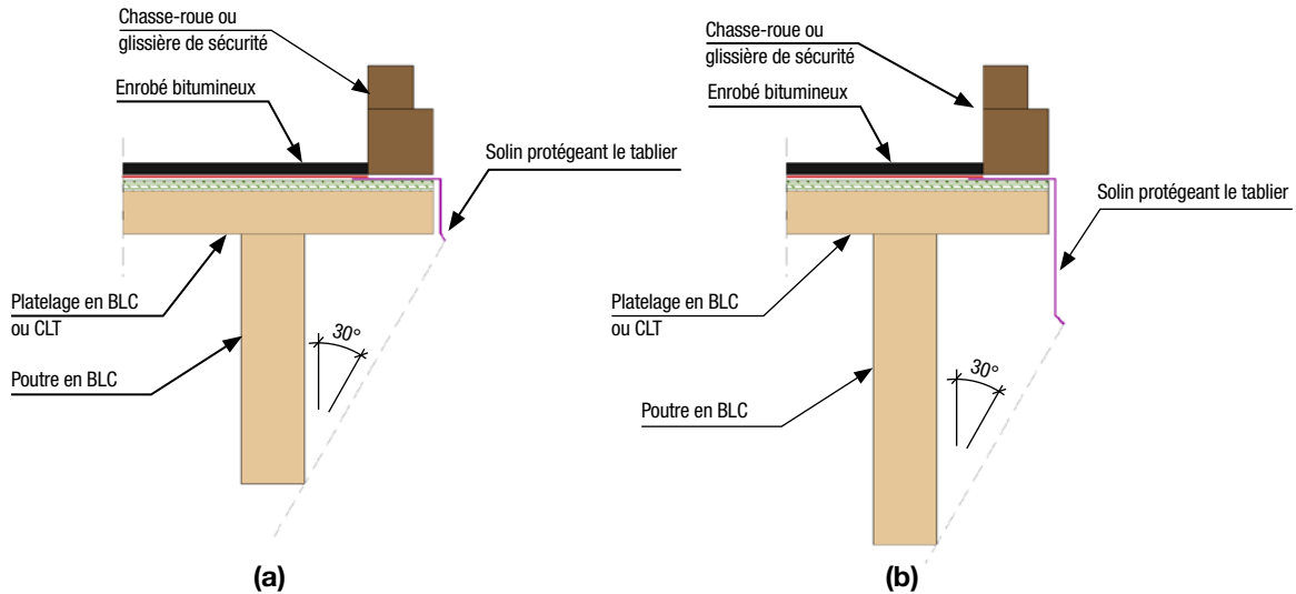
FIGURE 33 - Protection de la poutre de rive (a) par un platelage étanche surplombant la poutre avec un angle de 30° ou (b) par un solin plus long si le porte-à-faux est insuffisant
