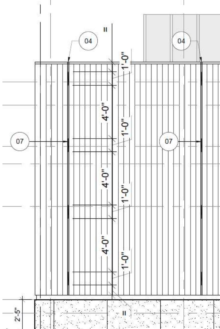
EXTRAIT ÉLEVATION EST
