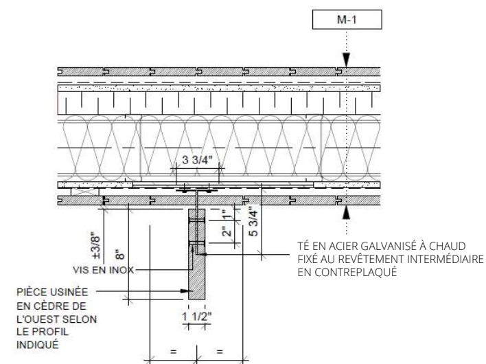
DÉTAIL TYPE - FIXATION DES PIÈCES DE BOIS DÉCORATIVES
