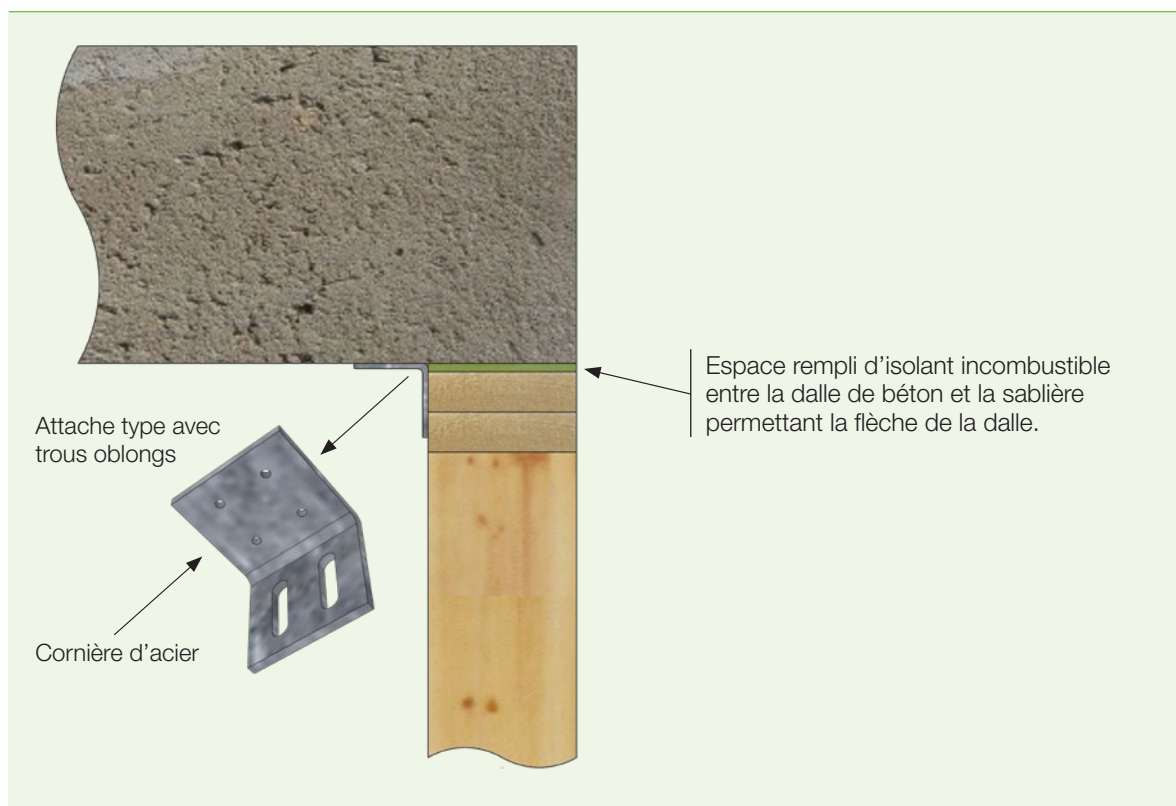
FIGURE 5 • Exemple d'attache de mur à la structure
