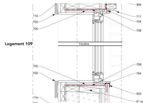
Coupe de mur montrant la position des fenêtres © Quinzhee
