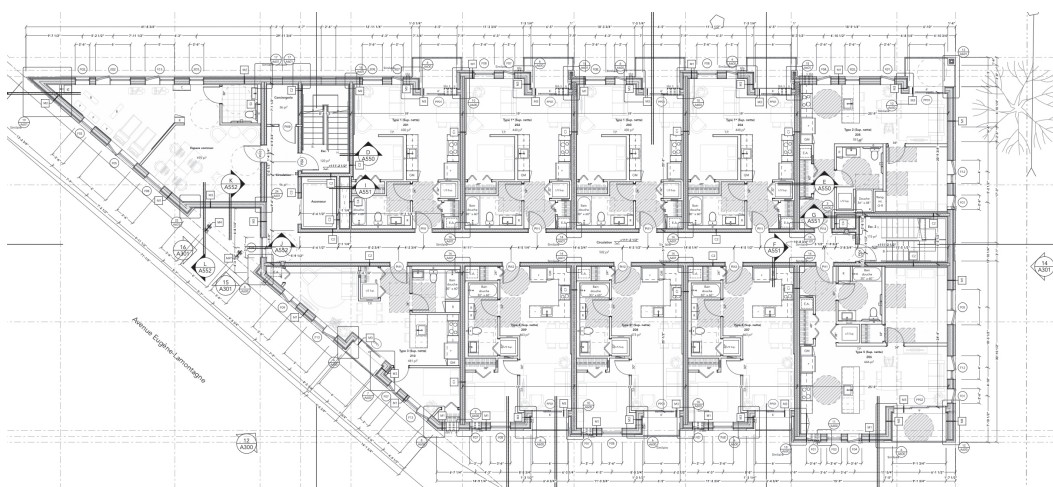
Plancher type du bâtiment Le Scandinave © Quinzhee
