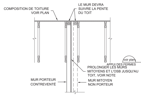
Fermes de toit et murs mitoyens © EQIP
