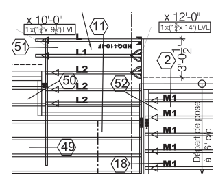
Plan des poutres en porte-à-faux soutenant le balcon à travers les poutres et l'enveloppe © Structures St-Joseph
