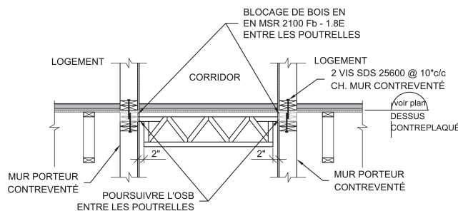
Disposition des poutres des planchers © EQIP
