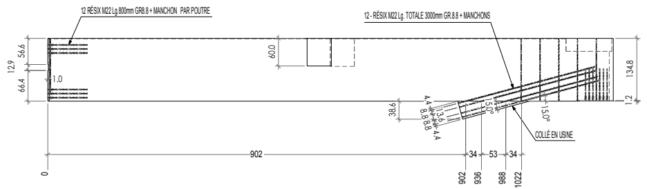
FIGURE 2 Connexion des tiges encollées aux poutres de la toiture © Structure Fusion
