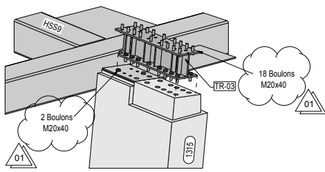
FIGURE 1 Connexion typique des tiges encollées aux colonnes © Structure Fusion
